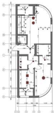
ПЛАН ОСВЕЩЕНИЯ М1000
