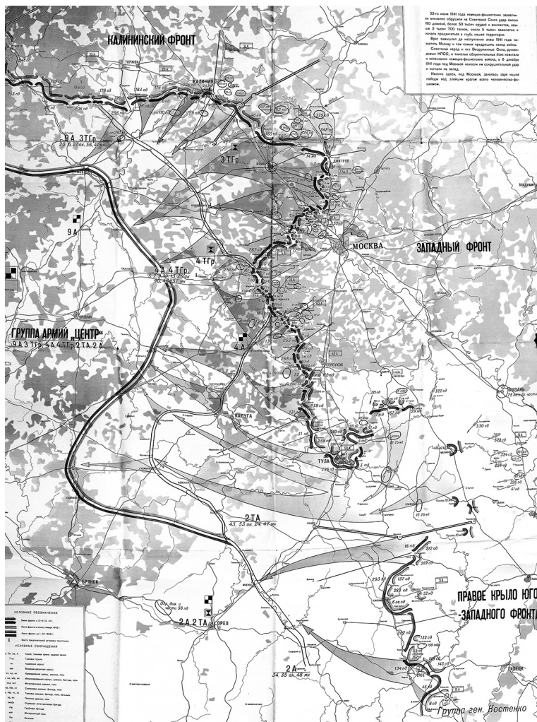
Рис. 5. Карта линии обороны и наступления частей РККА на Западном, Калининском и Юго-Западном фронтах. 1941 год.
