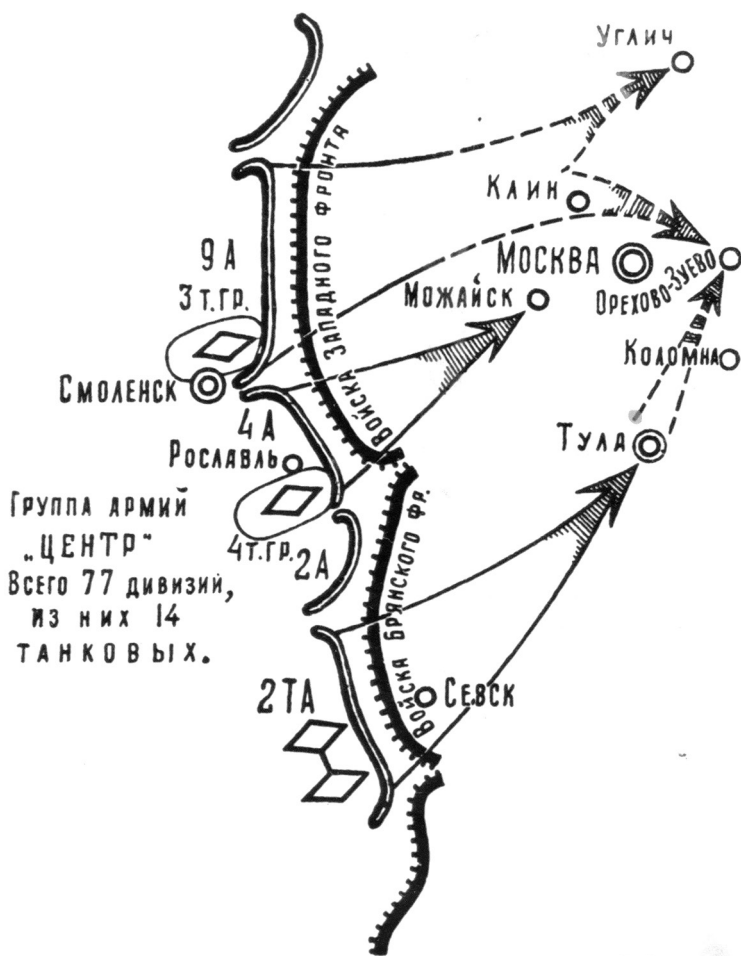
Рис. 4. Схематический план наступления немецко-фашистских войск на Брянском, Западном, Калининском и Юго-Западном фронтах в конце 1941 года; составлен после 1945 года.
